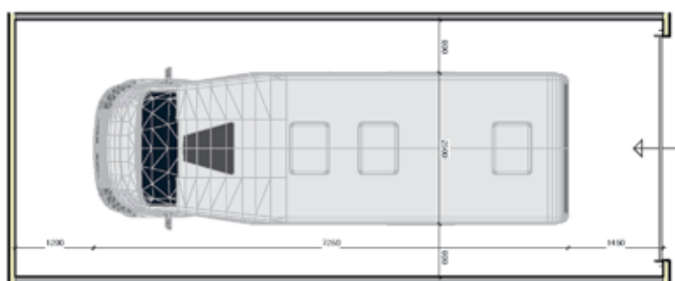
Bovenaanzicht camperbox
