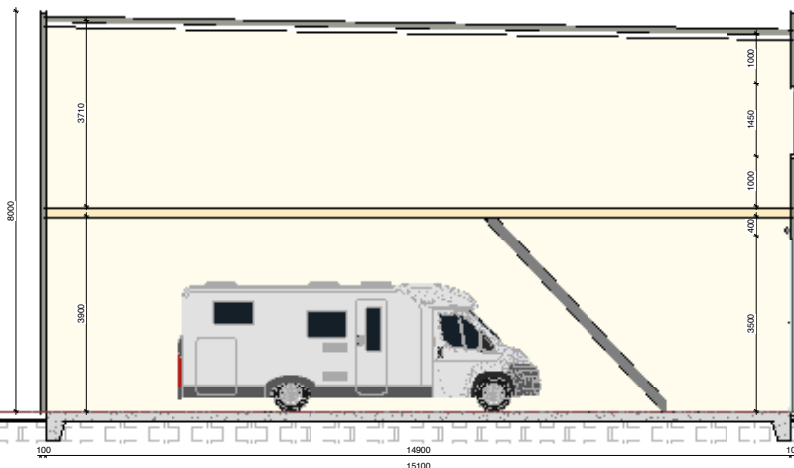
Doorsnede bedrijfsgebouw H - I
