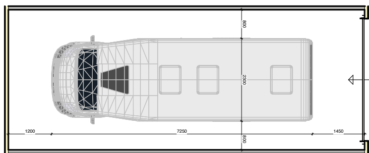
Bovenaanzicht camperbox
